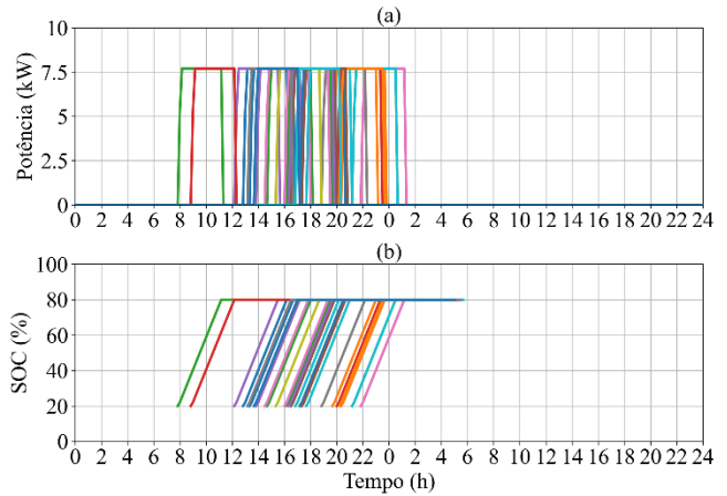
Fig. 6: Demanda dos veículos elétricos para recarga descoordenada e nível de penetração de 35%. a) Curva de recarga. b) Estado de carga.
