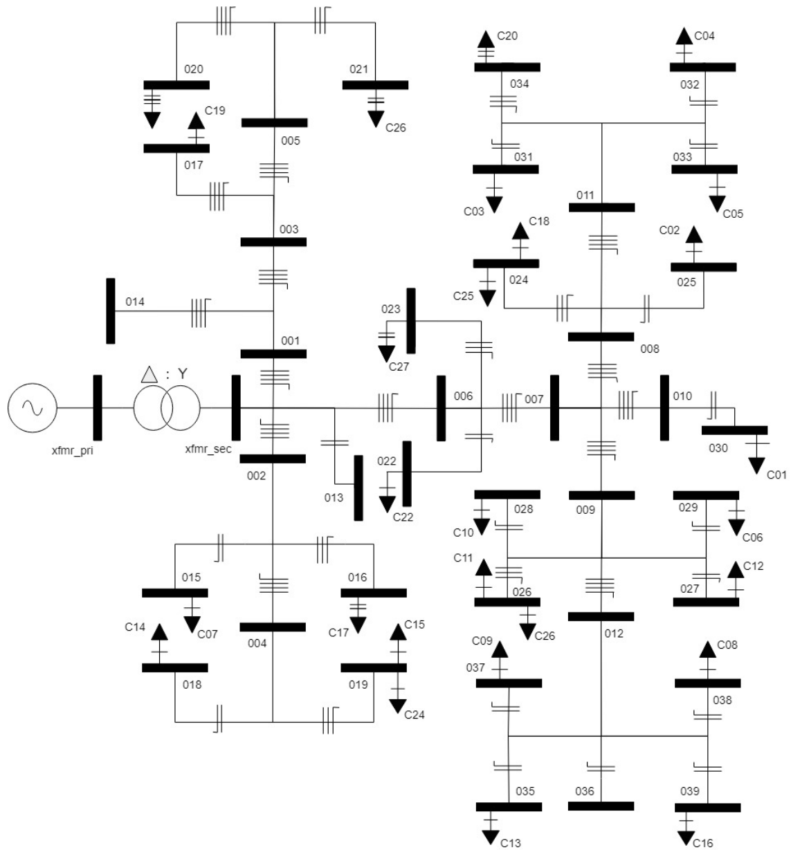
Figura A.1. Diagrama Unifilar do Caso de Estudo - Rede de distribuição Américo Brasiliense no estado de São Paulo
