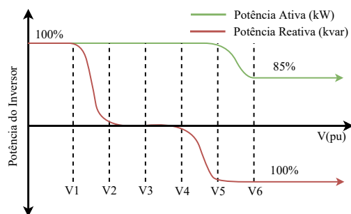
Figura 1. Curva ilustrativa da atuação dos controles Volt-Var e Volt-Watt diante da variação na tensão.
