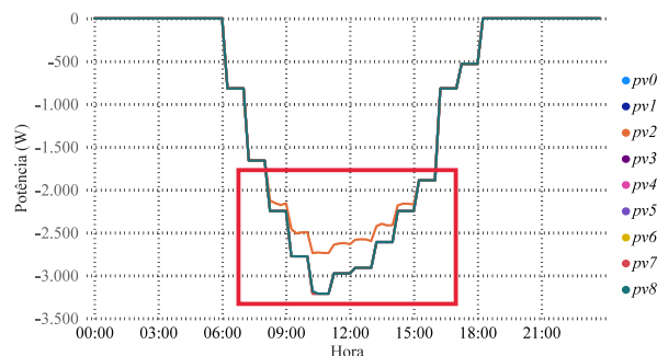
Figura 4. Potência ativa injetada pelos geradores: (a) Rede com PV e atuação do controle VV. (b) Rede com PV e atuação dos controles VV e VW
