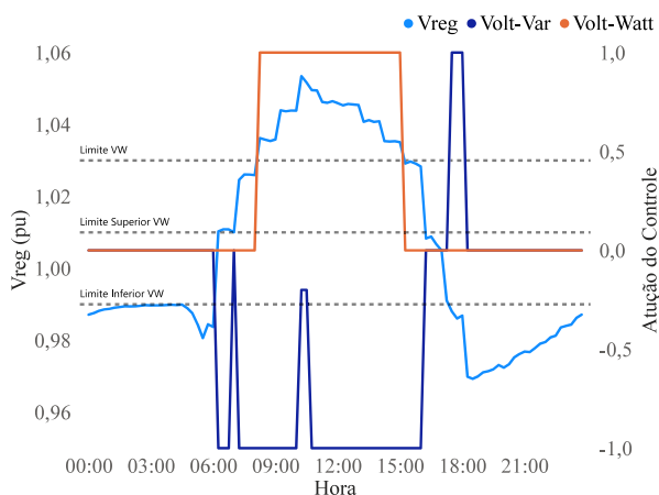
Figura 3. Atuação dos controles VV e VW frente a tensão de referência de uma geração fotovoltaica.
