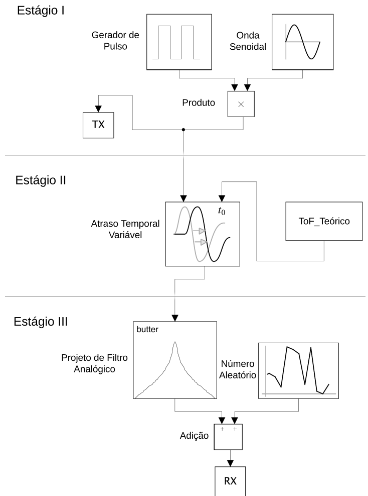
Figura 3. Modelo Simulink para comunicação entre TX e RX.
