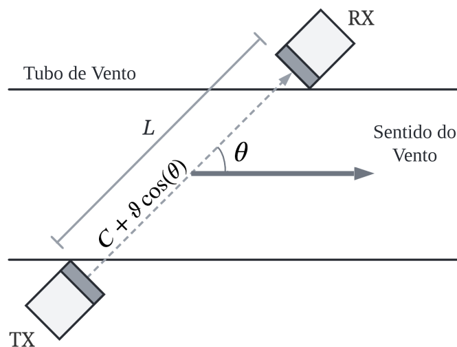
Figura 1. Configuração de estimativa da velocidade do vento utilizando transdutores ultrassônicos.
