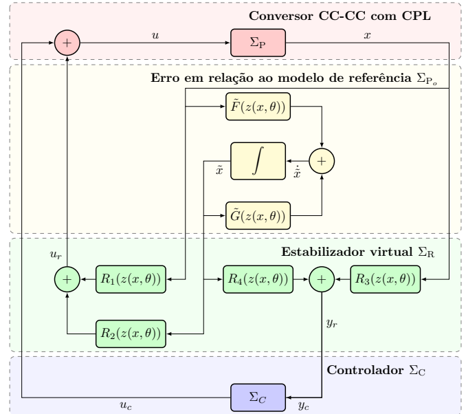
Figura 1. Sistema reconfigurado após a inserção do estabilizador reconfigurável virtual proposto na malha.
