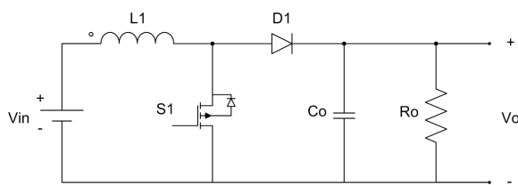
Figura 1. Conversor boost clássico c.c-c.c
