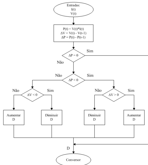
Figura 6. Fluxograma da técnica de MPPT-P&O
