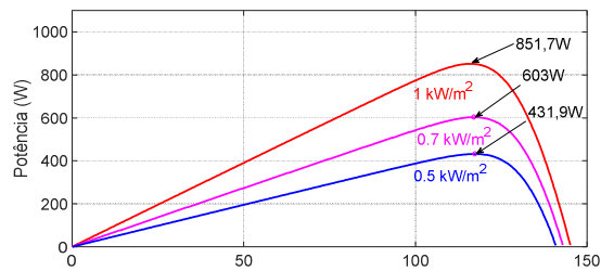
Figura 7. Potência disponível no sistema fotovoltaico considerando 1000W/m^2 , 700W/m^2 e 500W/m^2 .
