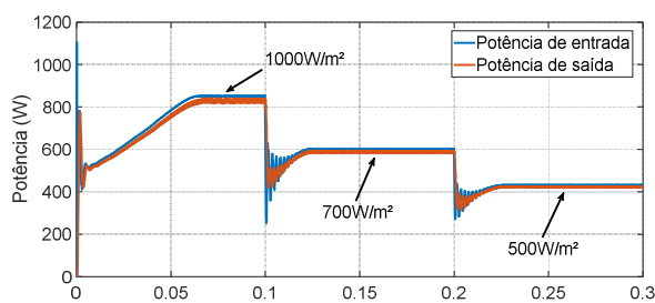
Figura 10. Potência drenada do sistema fotovoltaico e potência entregue a carga considerando o conversor boost convencional.
