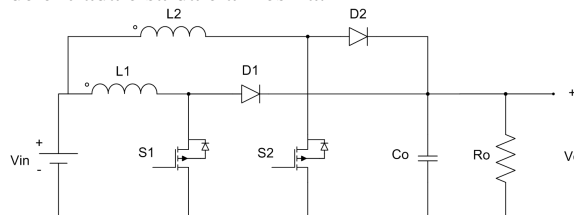
Figura 2. Conversor entrelaçado
