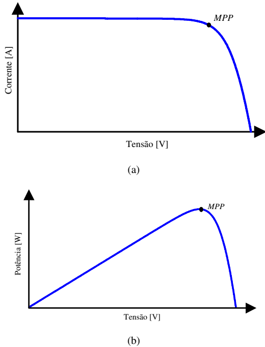
Figura 5. Curva característica da célula fotovoltaica (a) Tensão x Corrente (b) Tensão x Potência
