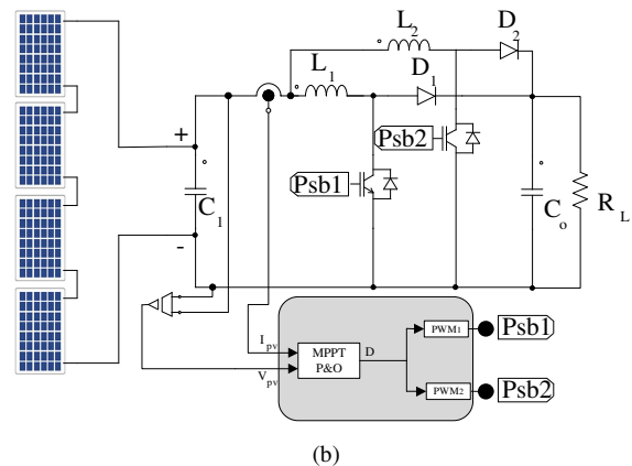
Figura 8. Sistema Fotovoltaico (a) com conversor boost convencional e (b) com boost interleaved
